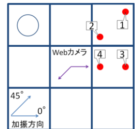
図-2 計測機器の設置位置
